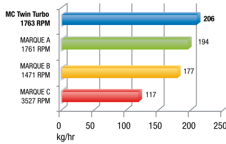
Vitesse de récupération en vapeur direct, kg/hr R22
