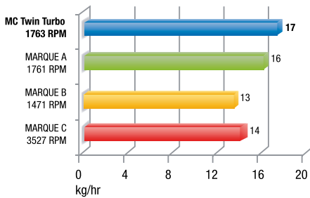
Vitesse de récupération en liquide direct, kg/hr R22
